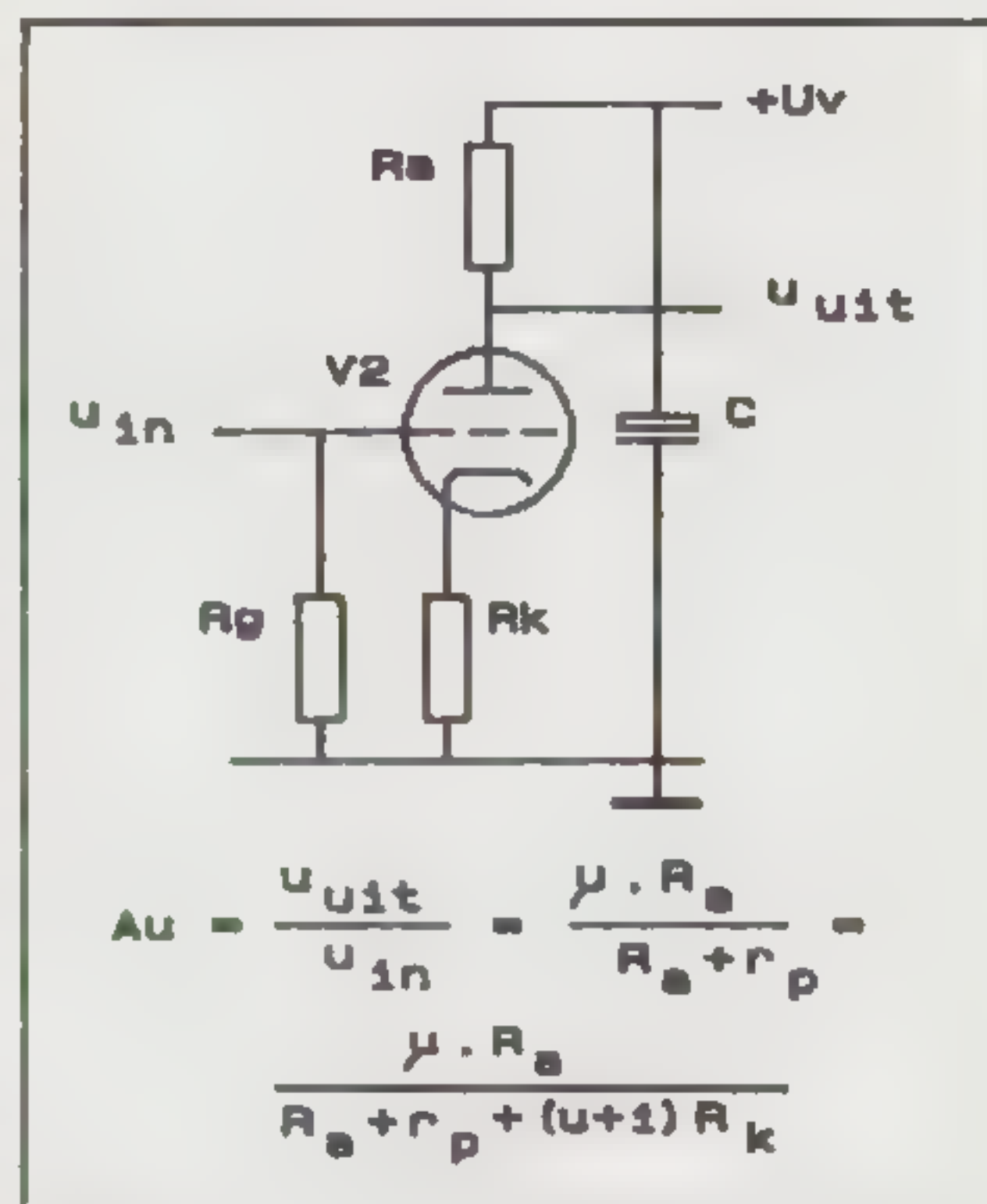
Figuur 10 Geaarde Kathode Schakeling
